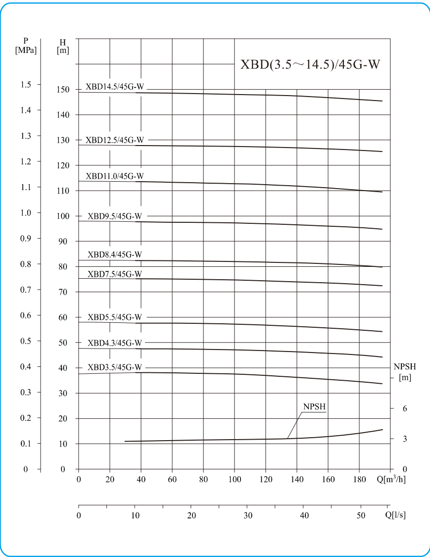
性能曲线
